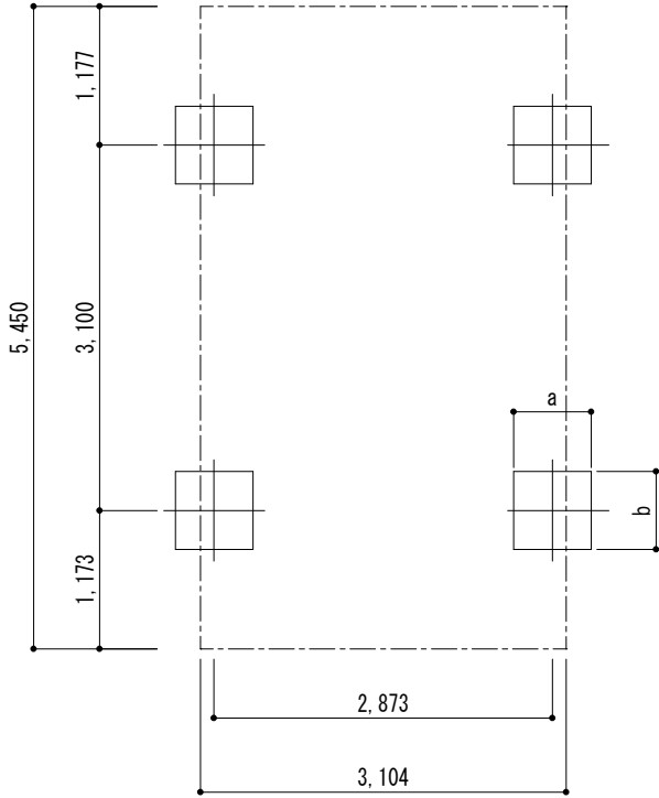
■ 基礎配置図
